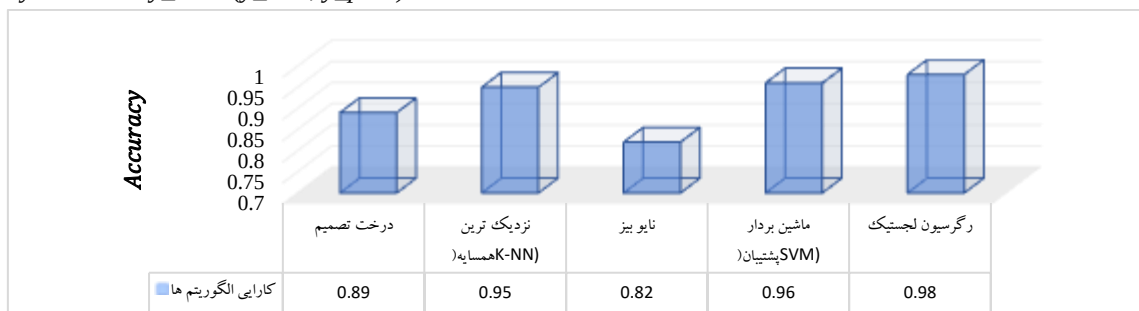
شکل ۵: مقایسه دقت طبقه‌بندی الگوریتم‌های مورد استفاده در پژوهش
